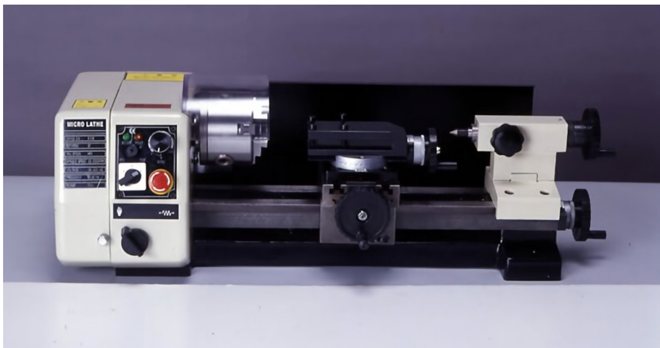
標準装備のトップスライドを取付けた状態
