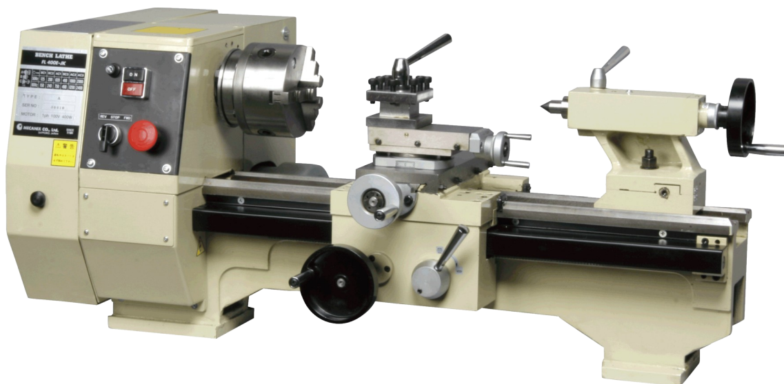
FL400E-JK(日立製モータを搭載)
