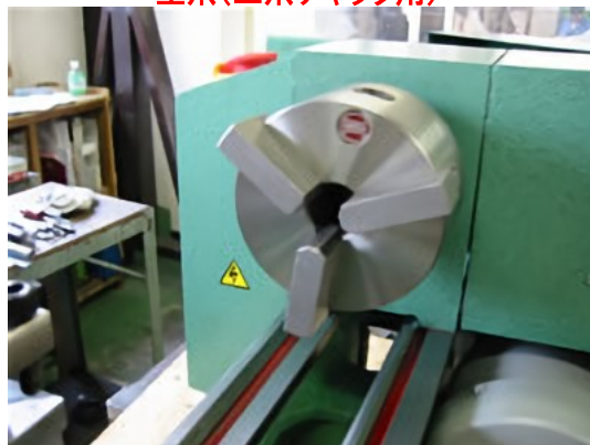
生爪(三爪チャック用)
