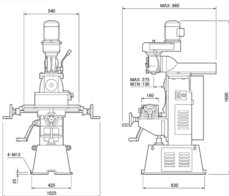
M40HVA 小型フライス盤 外観2面寸法図
