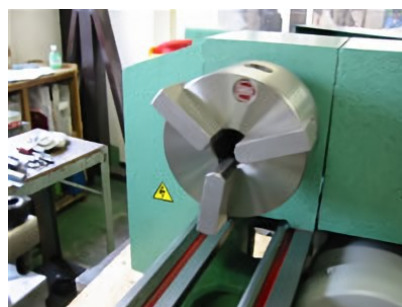
生爪(三爪チャック用) 生爪は成形可能な爪です。工作物の寸法や形状に合わせて成形できるため高精度のチャッキングが実現します。
