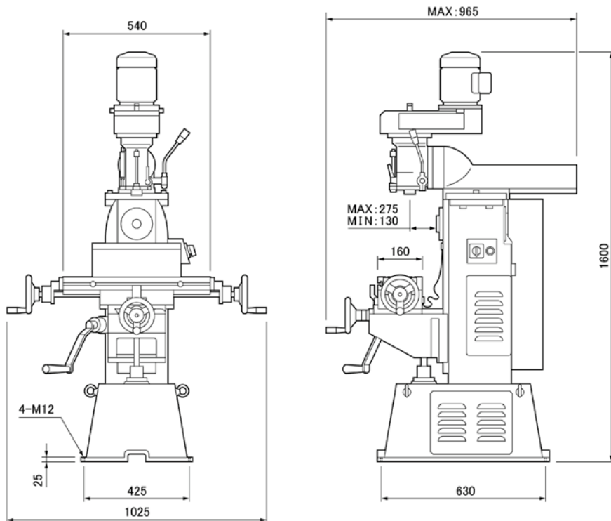
外観2面寸法図
