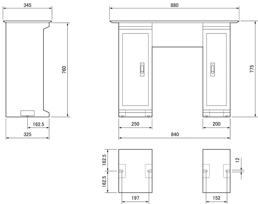
外観2面寸法図
